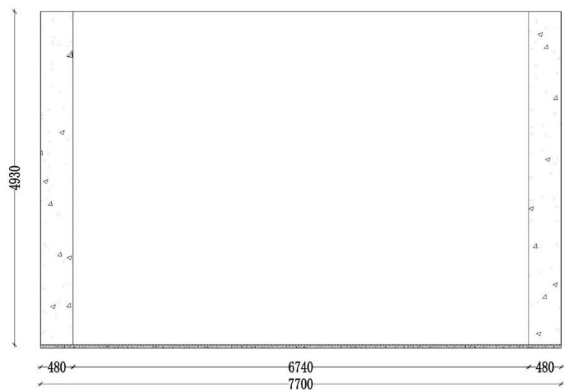
A03 LM-03 A03立面图
